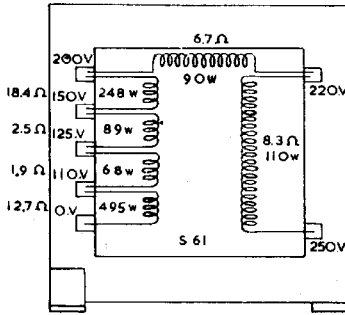
VOEDINGSTRAFO GK 512 74
