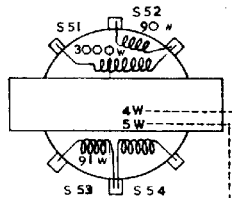
UITGANGSTRAFO GK 512 90 KY 505N 506N GK 512 80 KY 505 506
