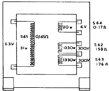
VOEDINGSTRAFO GK 512 74
